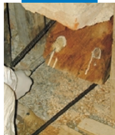
Applicazione di Mapewood Primer 100 mediante scovolino
